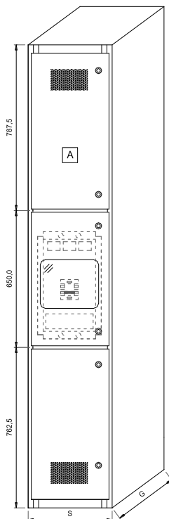
Widok elewacji:
