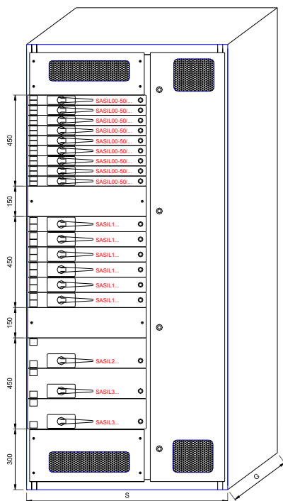
Widok elewacji:
